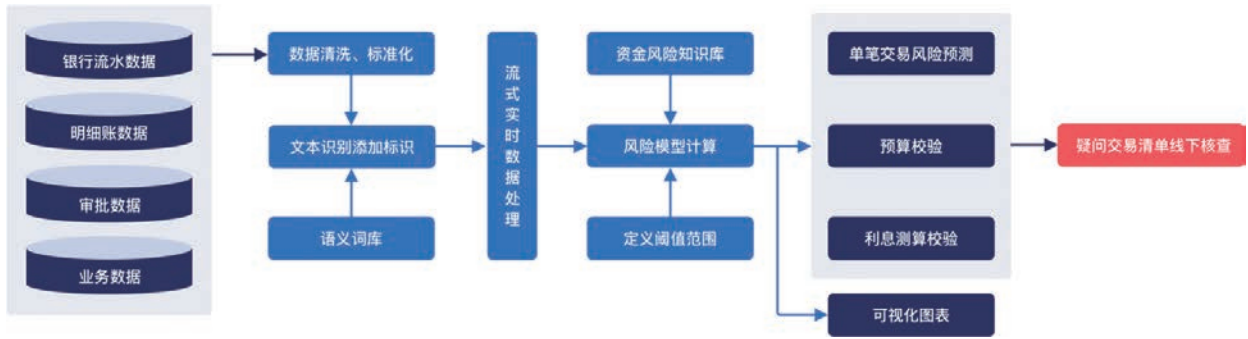
Figure 7 资金风险即时监控系统架构
